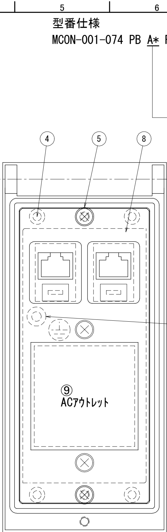
内部図
